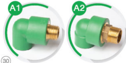
ข้องอ 90° เกลียวนอกทองเหลือง พีพีอาร์ MALE ELBOW 90° BRASS PP-R
